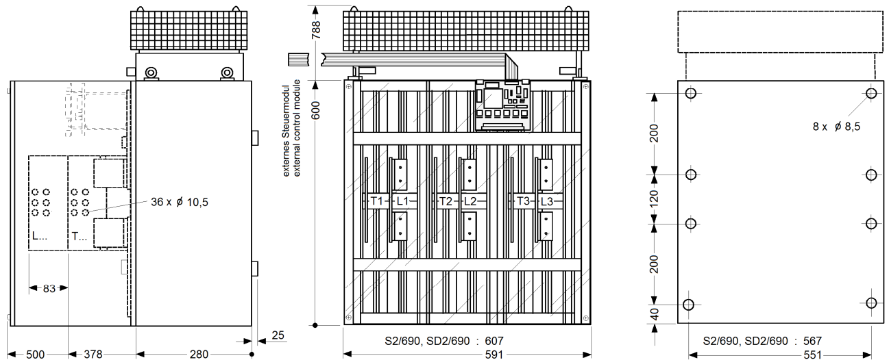
Maßbild / Outline drawing 6
