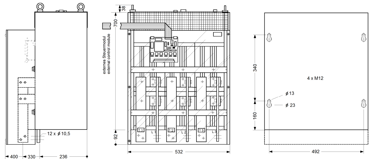
Maßbild / Outline drawing 5
